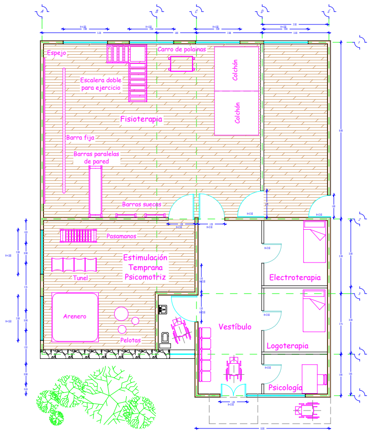
Planta Arquitectónica con muebles
